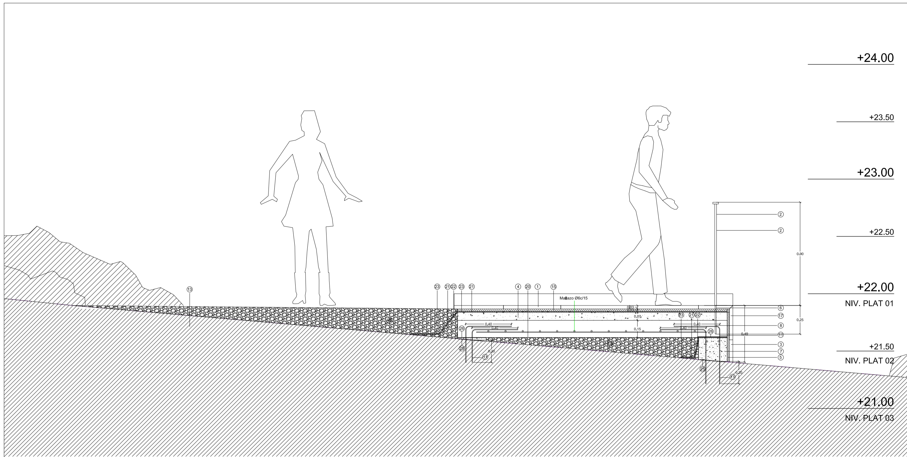
SECCIÓN TRANSVERSAL. ST1. E. 1/20 RANPA ACCESO
