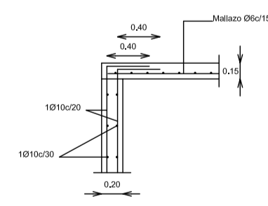
ARMADO MUROS Y CONEXIÓN MUROS - SOLERA E:1/50
