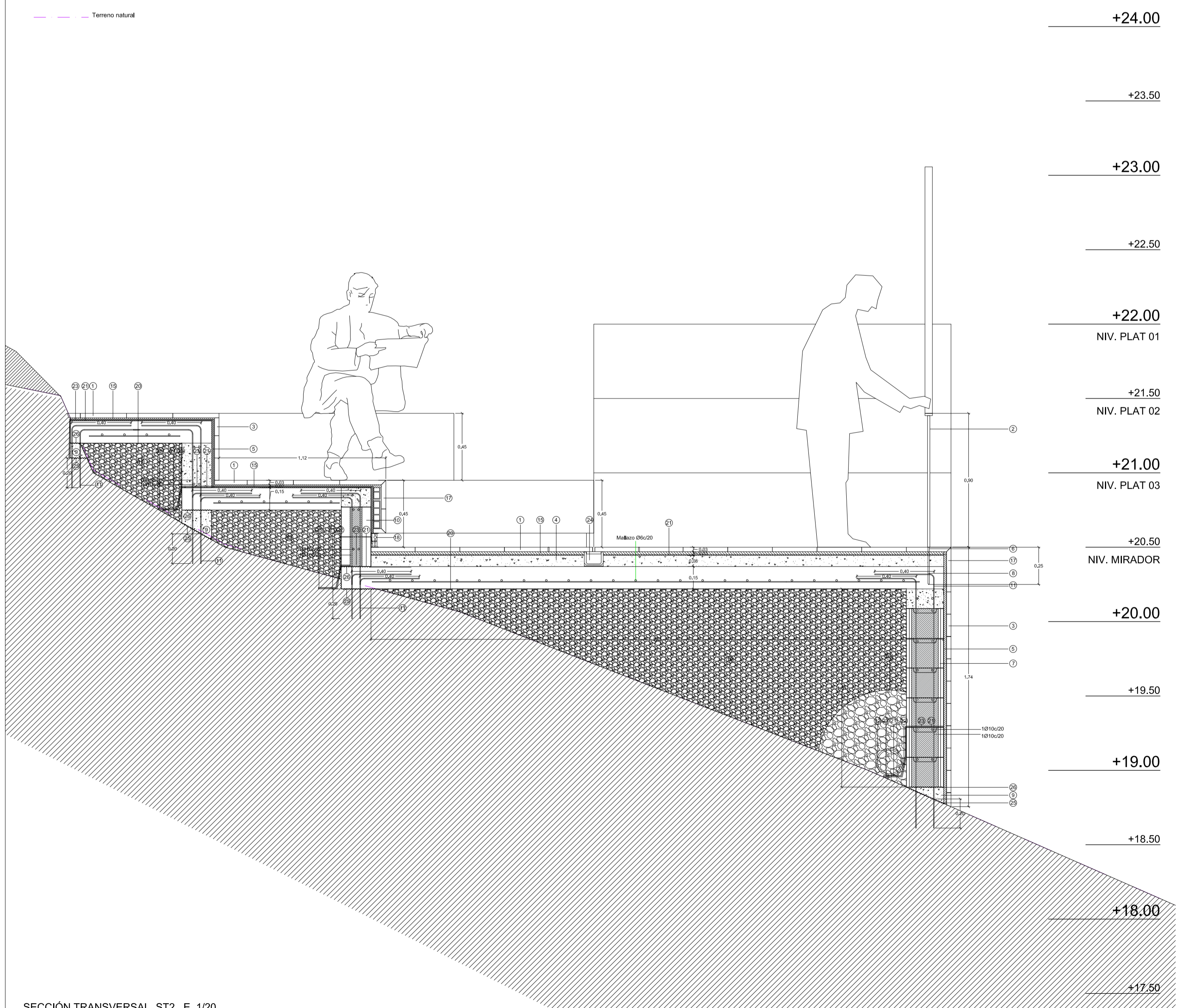
SECCIÓN TRANSVERSAL. ST2. E. 1/20 PLATAFORMA MIRADOR-BANCOS
